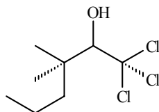
1,1,1-trichloro-3,3-dimethylhexan-2-ol
