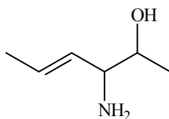
(4E)-3-aminohex-4-en-2-ol
