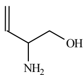
2-amino-3-buten-1-ol
